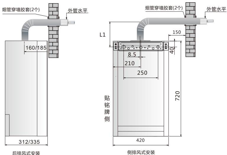
烟道安装示意图
